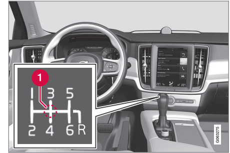
Řadicí páka a schéma řazení - přehled.
