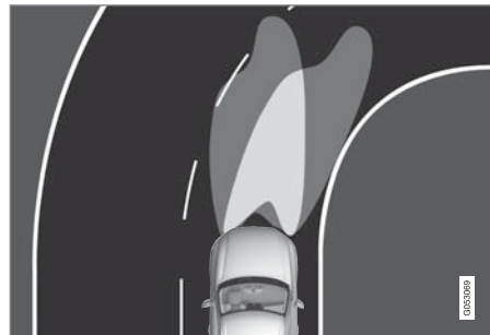
頭燈燈照模式功能關閉 (左) 與啟動 (右) 的情況。
