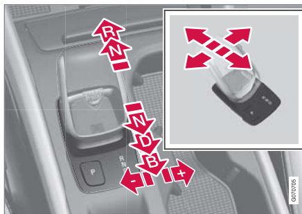
排檔桿和檔位概覽。
