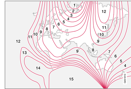
Mágneses zónák
