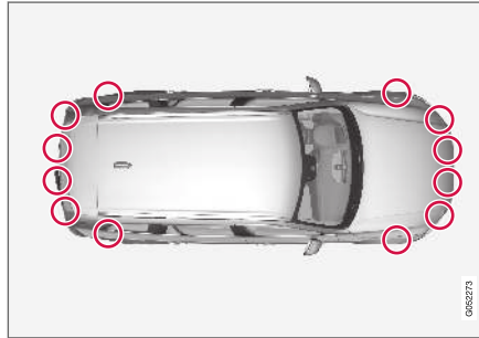
A parkolőérzékelők elhelyezkedése 132 .
