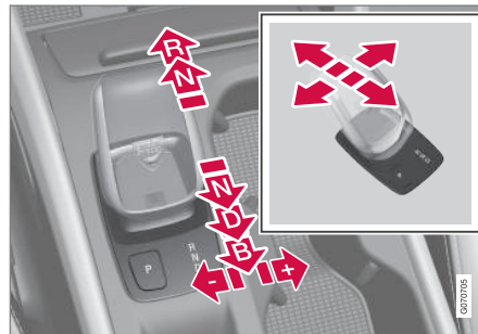
A fokozatválasztó kar és a fokozathelyezetek áttekintése.
