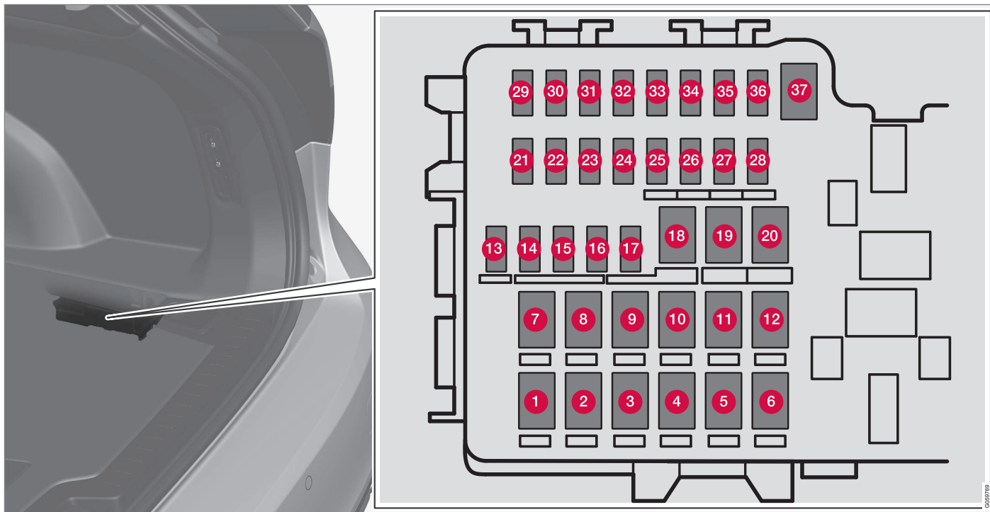
Centralka elektryczna znajduje się po prawej stronie.
