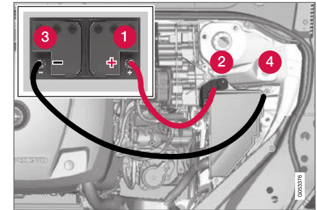
Point de charge pour l'aide au démarrage pour la voiture.
