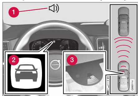
Elementy układu 67 .
