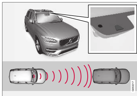
Umiejscowienie modułu radarowego 66 .
