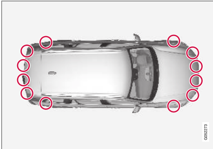
Lokalizacja czujników parkowania 109 .
