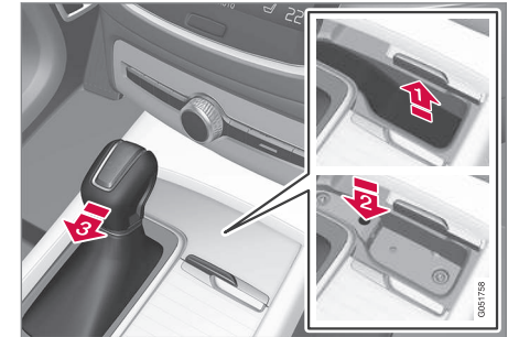
Prezentacja dużej dźwigni zmiany biegów.
