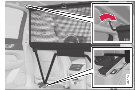
Első rögzítés.
