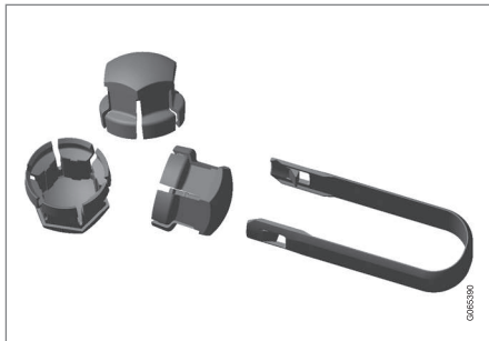
Verktyg för borttagning av plashattar på hjulskruvarna.
