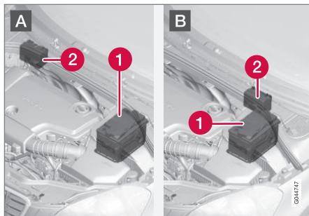
A: Automašīna ar stūri kreisajā pusē. B: Automašīna ar stūri labajā pusē. (1). Startera akumulators 17 (2). Atbalsta akumulators.
