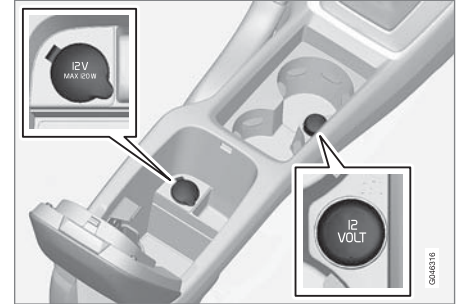
مقيس ١٢ فولت في الكونسول النفق، المقعد الأمامي.
