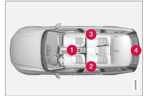
Umiejscowienie anten.
