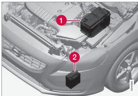
(1) Startbatteri 13 (2) Stödbatteri
