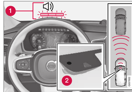
Avertissement de collision sur le pare-brise 50 .
