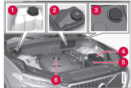
엔진룸의 외관은 모델 및 엔진 종류에 따라 다를 수 있습니다.
