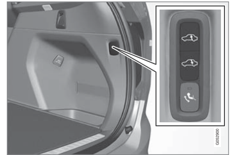
車身後段降低/升高的控制裝置
