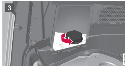
Разширителен резервоар за охлаждайна течност
