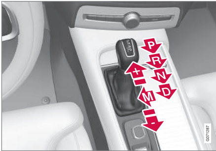
Преглед на големия скоростен лост и положението на предавките.
