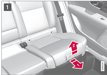
1 핸들을 앞쪽과 위쪽으로 당겨 시트 쿠션을 해제합니다.
