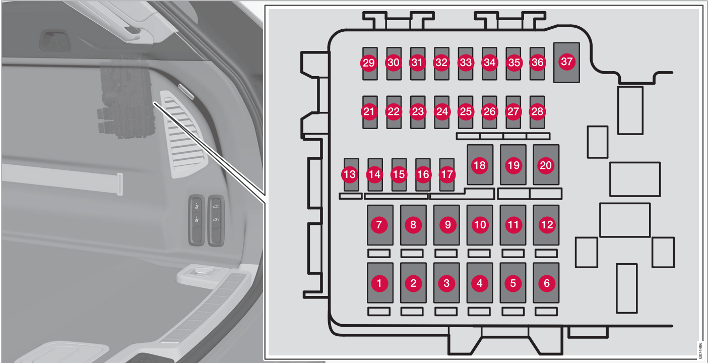
중앙 전기장치는 우측에 있습니다.
