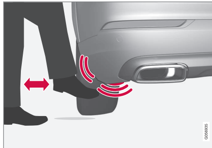
유효한 감지기 작동 구역 내의 차는 동작.
