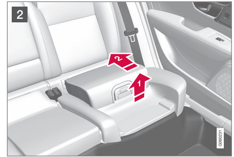
2 시트 쿠션의 앞쪽 가장자리를 들어올려 등받이 쪽으로 밀어 고정합니다.
