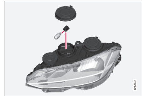
좌측 전조등.
