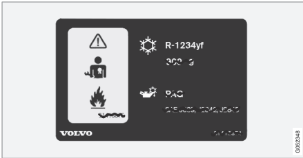
2 냉매 R1234yf를 사용하는 차량의 A/C 시스템 스티커.
