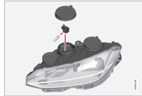
좌측 전조등.
