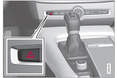
비상등 버튼.
