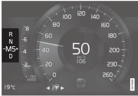
소형 기어 선택터용 8인치 운전자 화면의 기어 변속 표시등.
