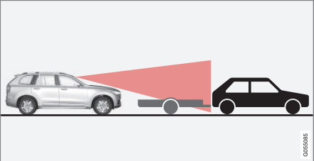
레이더 음영 지대에 있는 낮은 트레일러
