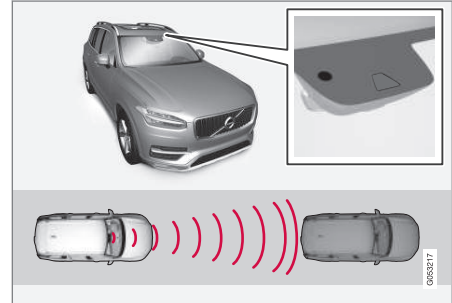
카메라 및 레이더 유닛은 앞차와의 간격을 측정합니다.
