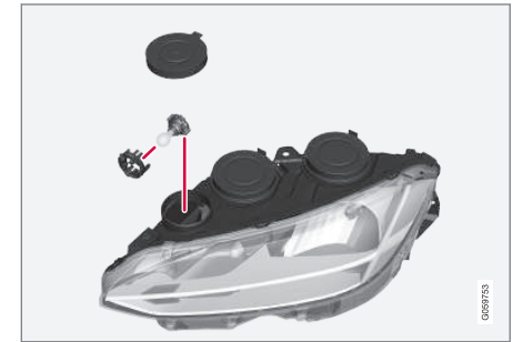
Ляв преден фар.
