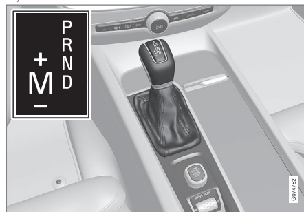
Pregled velike prestavne ročice in vzorca prestav na voznikovem zaslonu.
