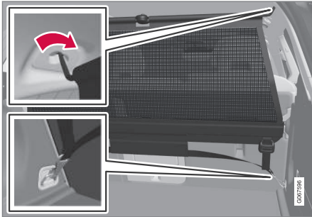
Заден монтаж.
