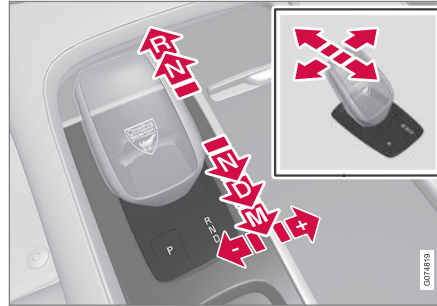
Преглед на малкия скоростен лост и положението на предавките.
