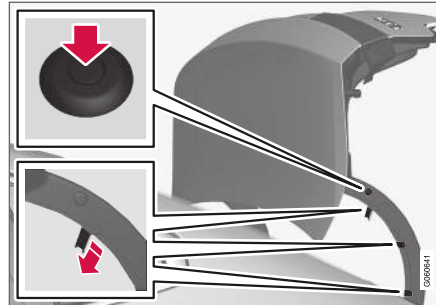
Plastikowa osłona zawiasu jest zamocowana za pomocą plastikowego nitu i trzech zaczepów.
