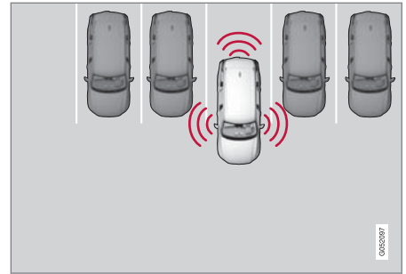
평행 주차 중의 위치 추적 원리.
