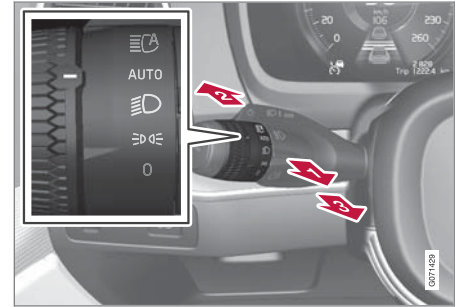
회전 링이 있는 스티어링휠 레버 스위치
