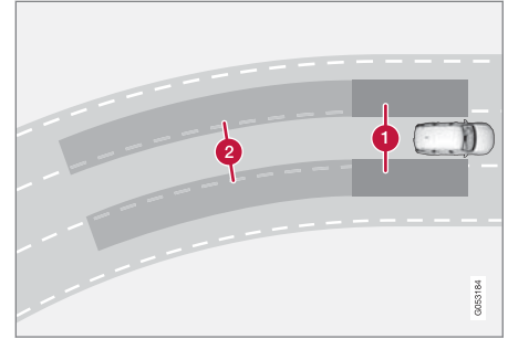
BLIS의 작동 원리
