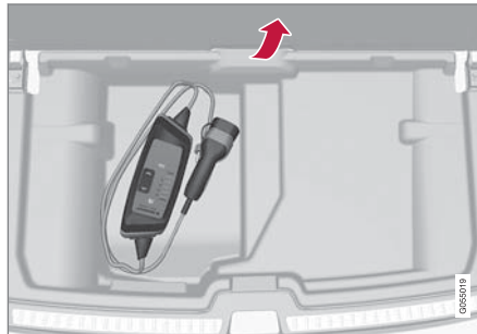
충전 케이블은 트렁크의 바닥 해치 아래의 보관함에 있습니다.
