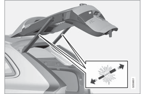
전동 테일게이트용 사전 장력 조정 스프링.
