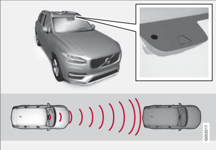
카메라 및 레이더 유닛은 앞차와의 간격을 측정합니다.
