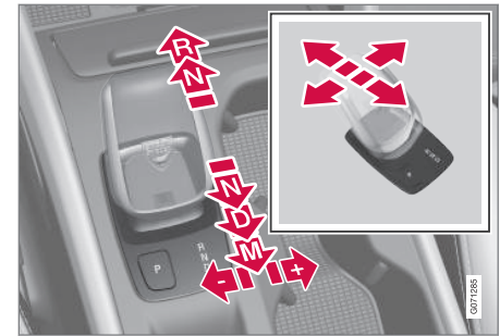
Vue d'ensemble du petit levier de vitesses et des positions de rapport.
