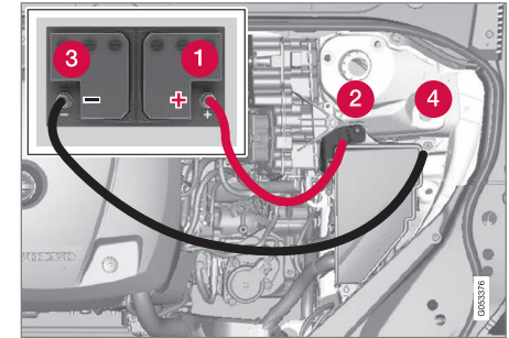
Points de raccordement du câble volant.
