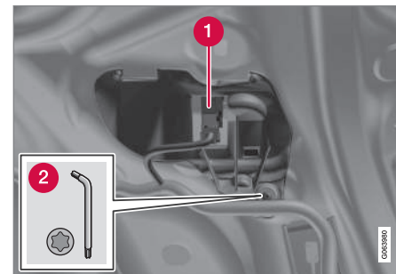
Obudowa światła z pokrywą po prawej stronie.
