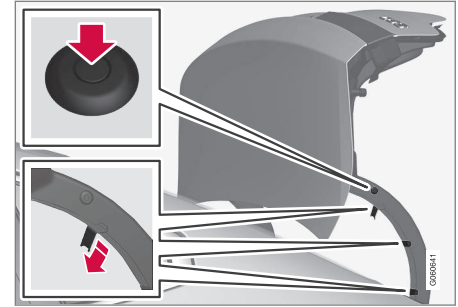
Plastikowa osłona zawiasu jest zamocowana za pomocą plastikowego nitu i trzech zaczepów.
