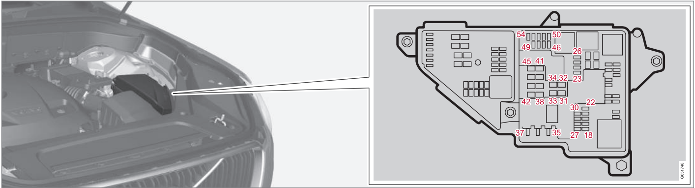
Section arrière de la centrale électrique avec les fusibles 18 à 54.
